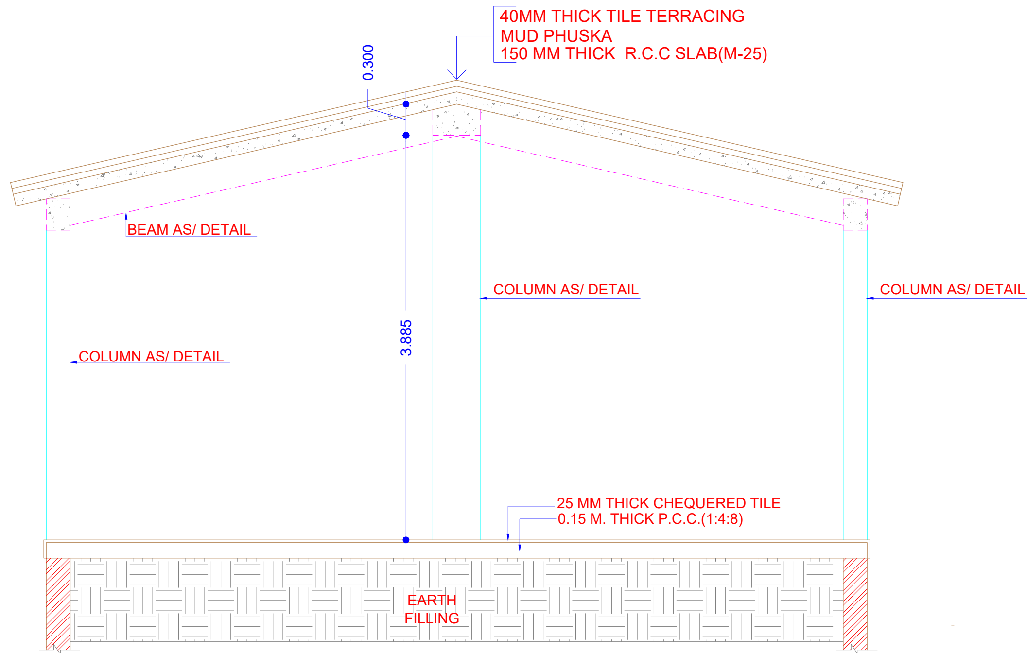
SECTION A-B
